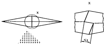
图 2 压头锥顶交线 (示意图)
