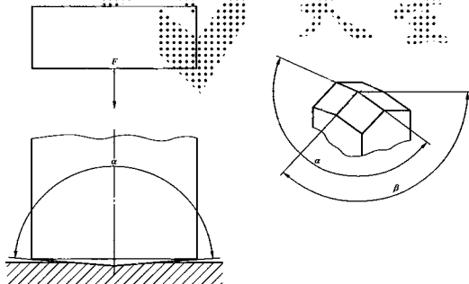
图 1 试验原理和压头几何形状
