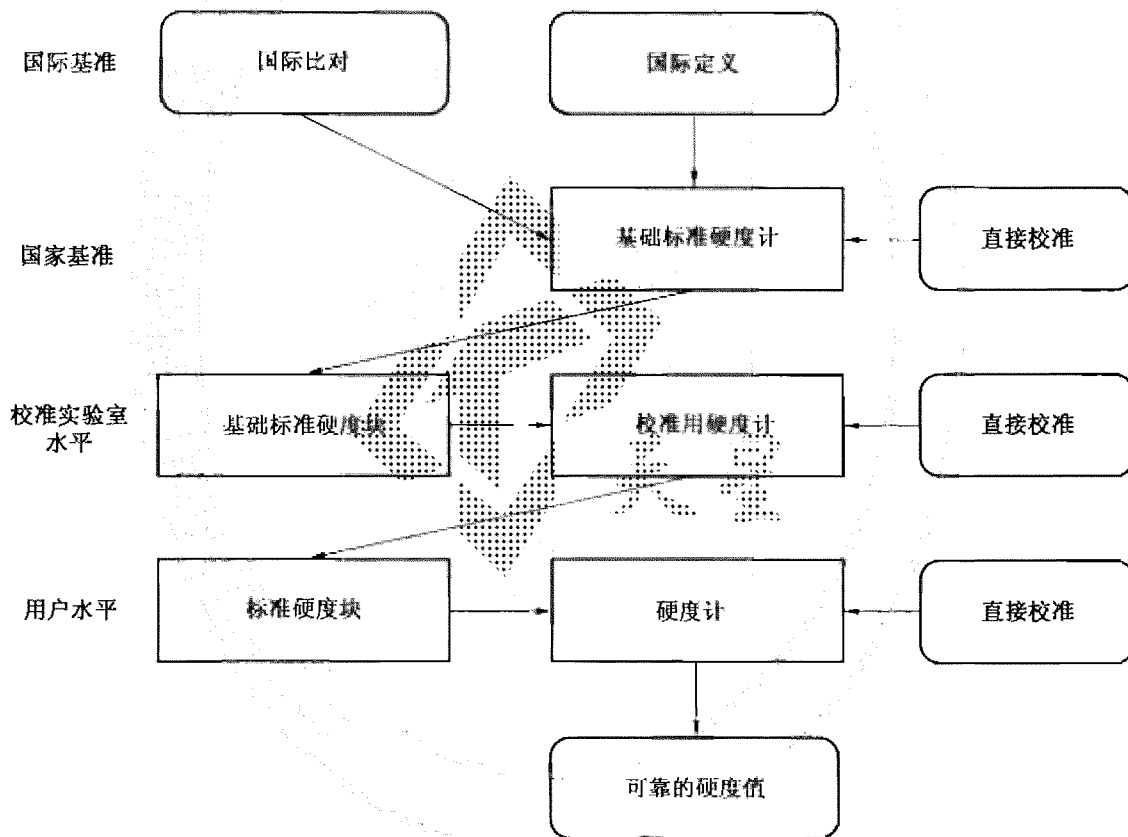
图 D.1 硬度标尺的定义和量值传递图
