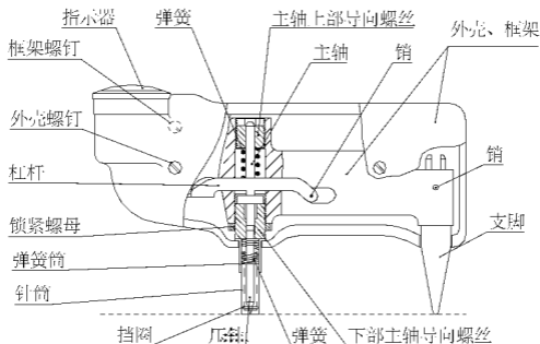
图2 巴氏硬度计结构图
